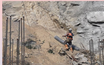
鋼線網鋪設
