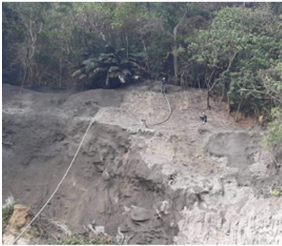
上方邊坡噴漿作業
